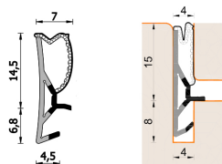
A 255 STP BOB DIR Per serramenti in legno
