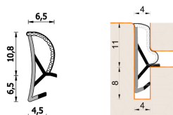
A 254 STP BOB DIR Per serramenti in legno
