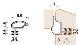
A 498 STP BOB Per serramenti in legno
